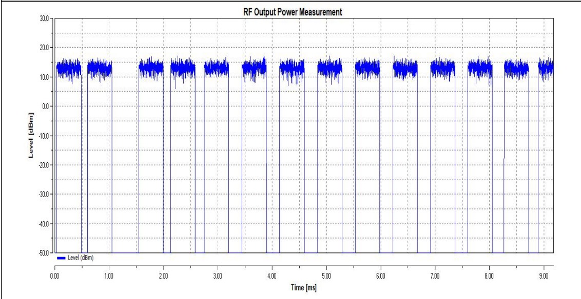
LTNV_11AX20SISO_Ant1_2472
