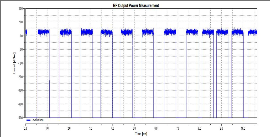
HTNV_11AX20SISO_Ant1_2412
