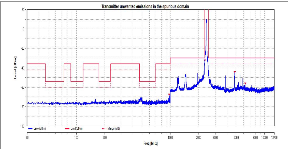
11AX40SISO_Ant1_2462
