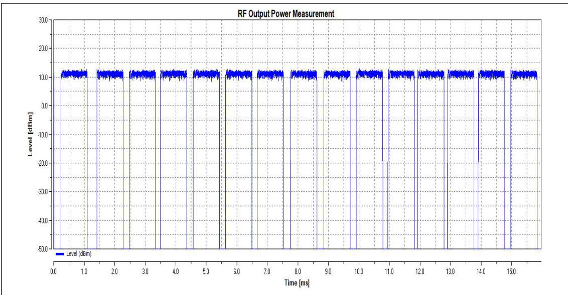
NTVN_11G_Ant1_2412
