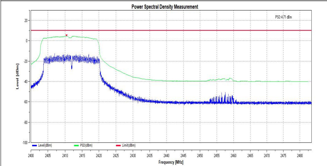
11G_Ant1_2442
