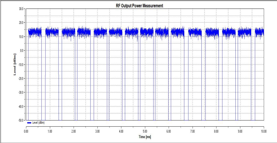
LTNV_11N20SISO_Ant1_2472
