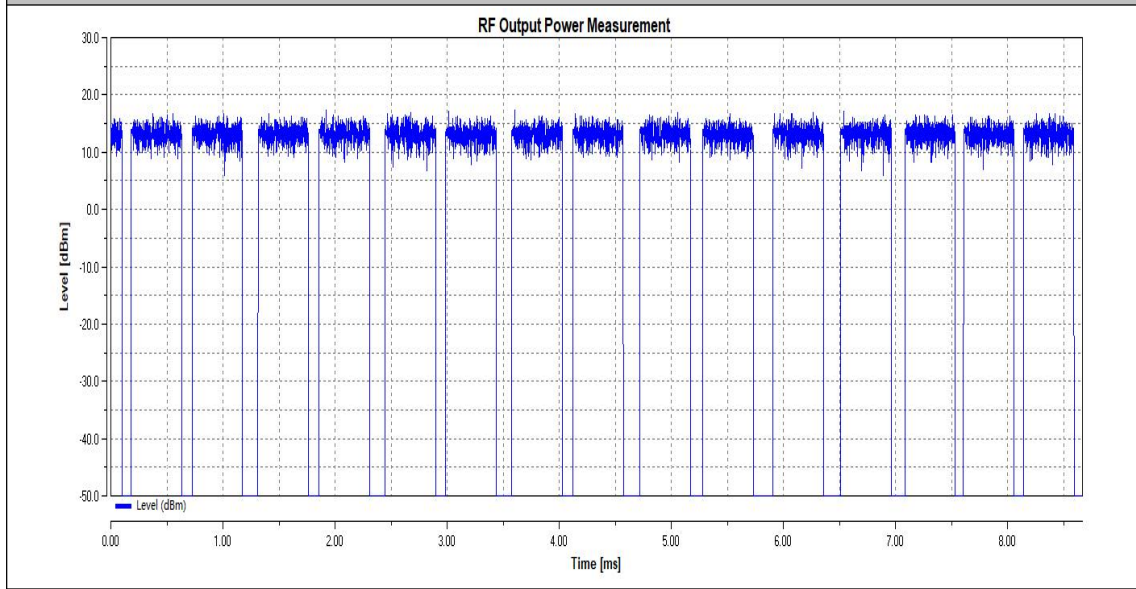
NTNV_11AX20SISO_Ant1_2472
