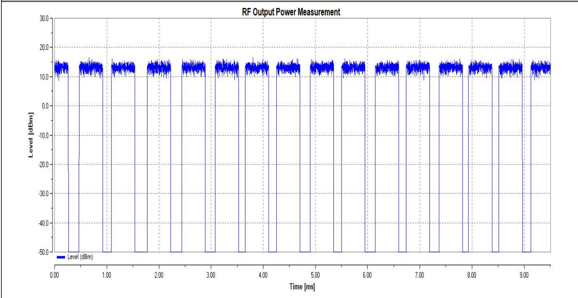
NTNV_11AX40SISO_Ant1_2442
