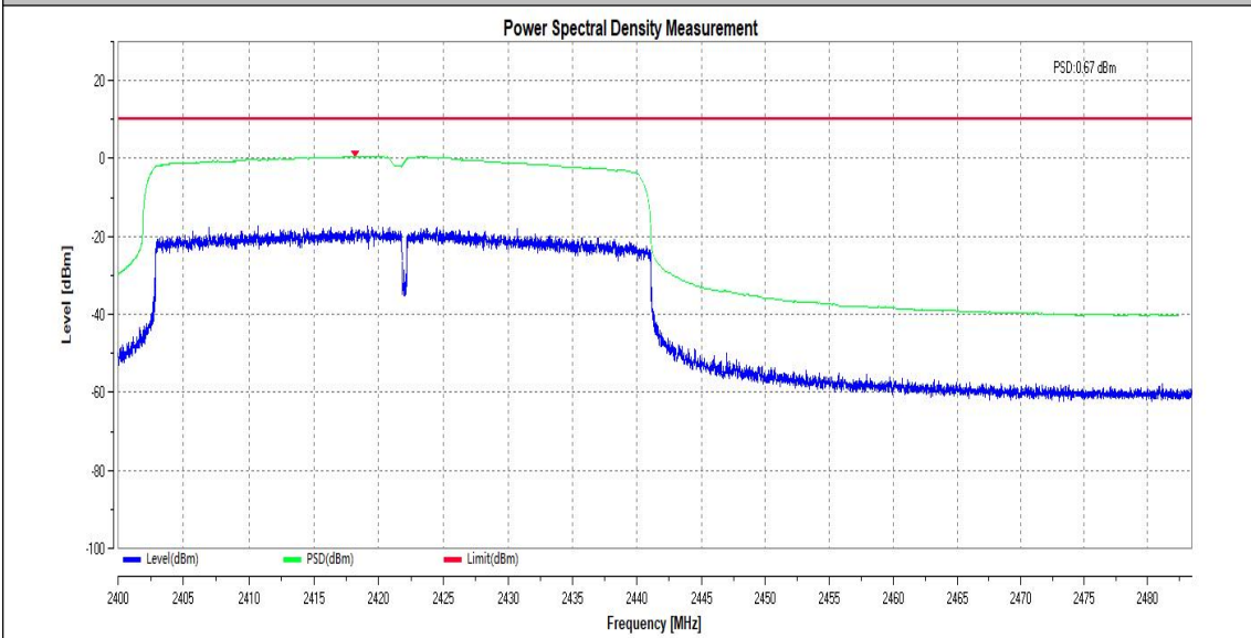
11AX40SISO_Ant1_2442
