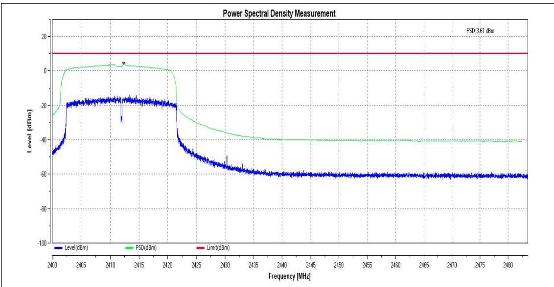
11AX20SISO_Ant1_2442
