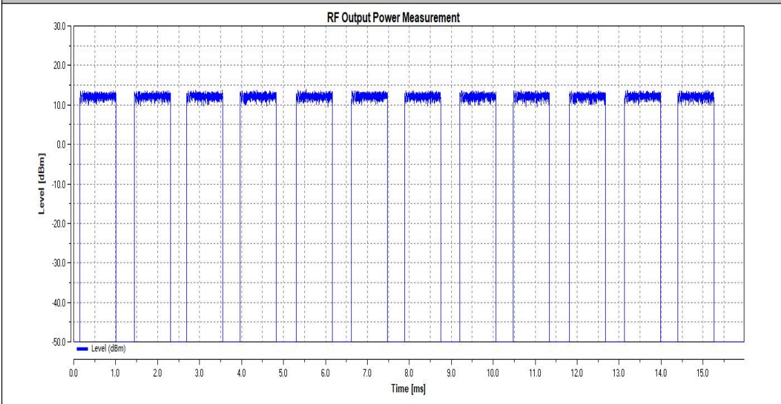
LTNV_11B_Ant1_2472
