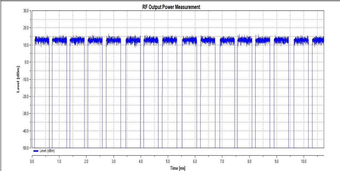
NTNV_11AX20SISO_Ant1_2412
