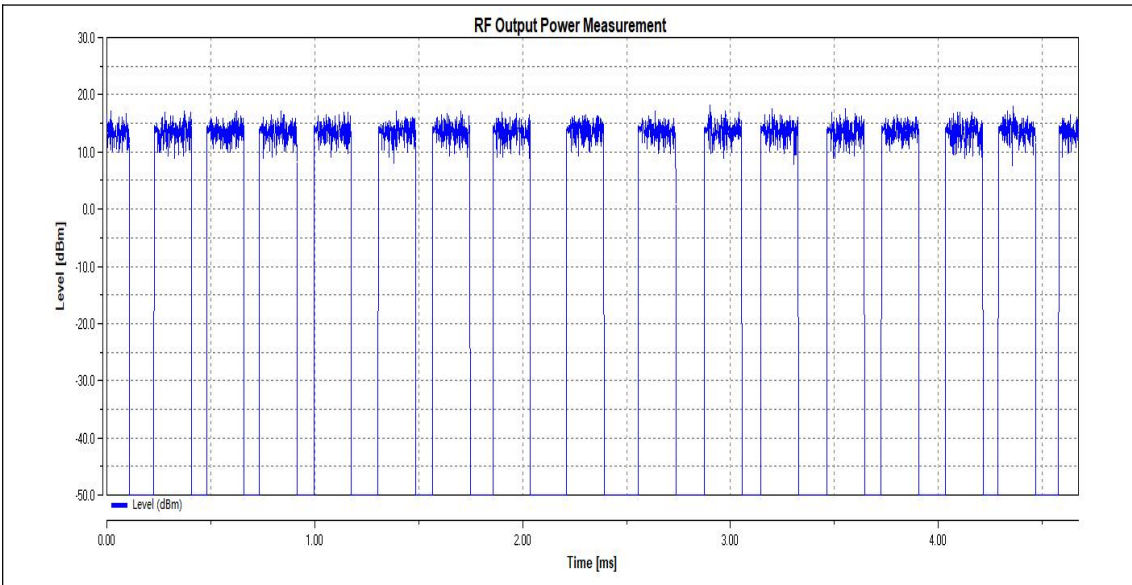
LTNV_11G_Ant1_2472
