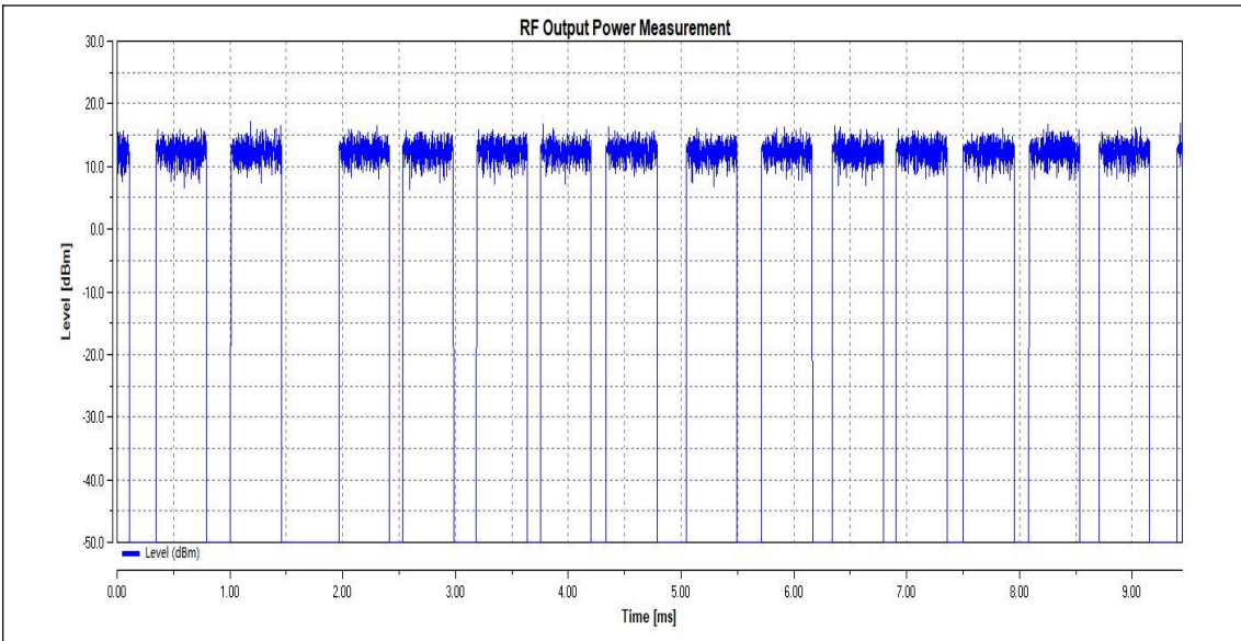
HTNV_11AX40SISO_Ant1_2422
