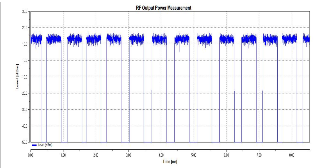
HTNV_11AX20SISO_Ant1_2442
