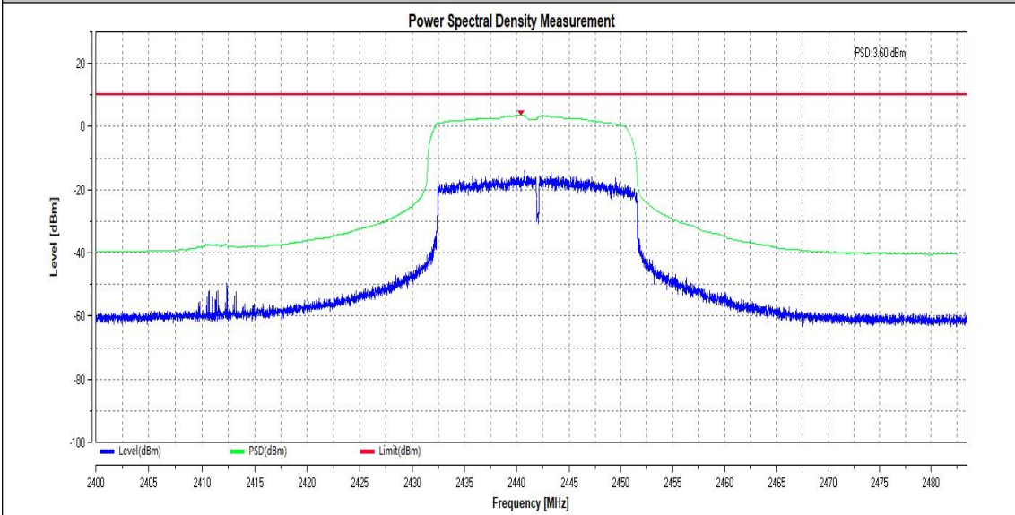
11AX20SISO_Ant1_2472
