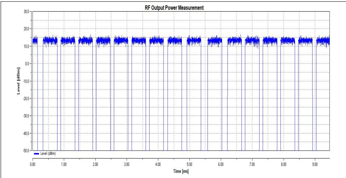
NTNV_11AX40SISO_Ant1_2462
