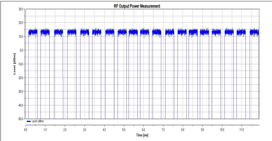
LTNV_11AX40SISO_Ant1_2462
