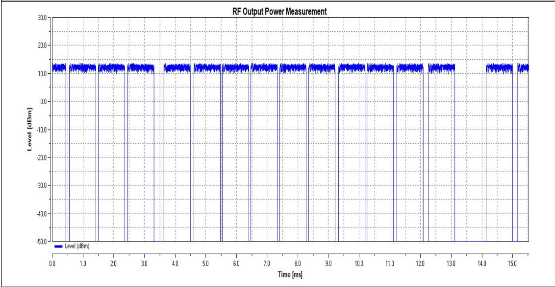
HTNV_11B_Ant1_2472
