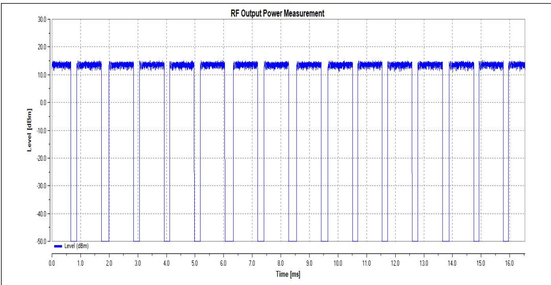
LTNV_11B_Ant1_2442
