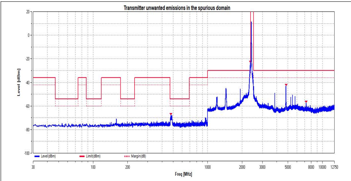
11N20SISO_Ant1_2472
