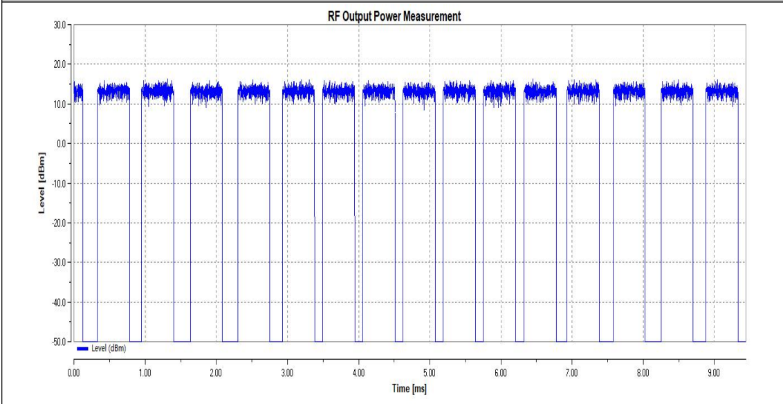
LTNV_11AX40SISO_Ant1_2442
