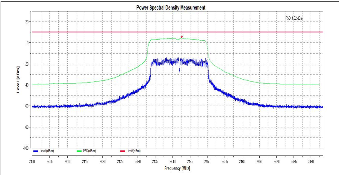
11G_Ant1_2472
