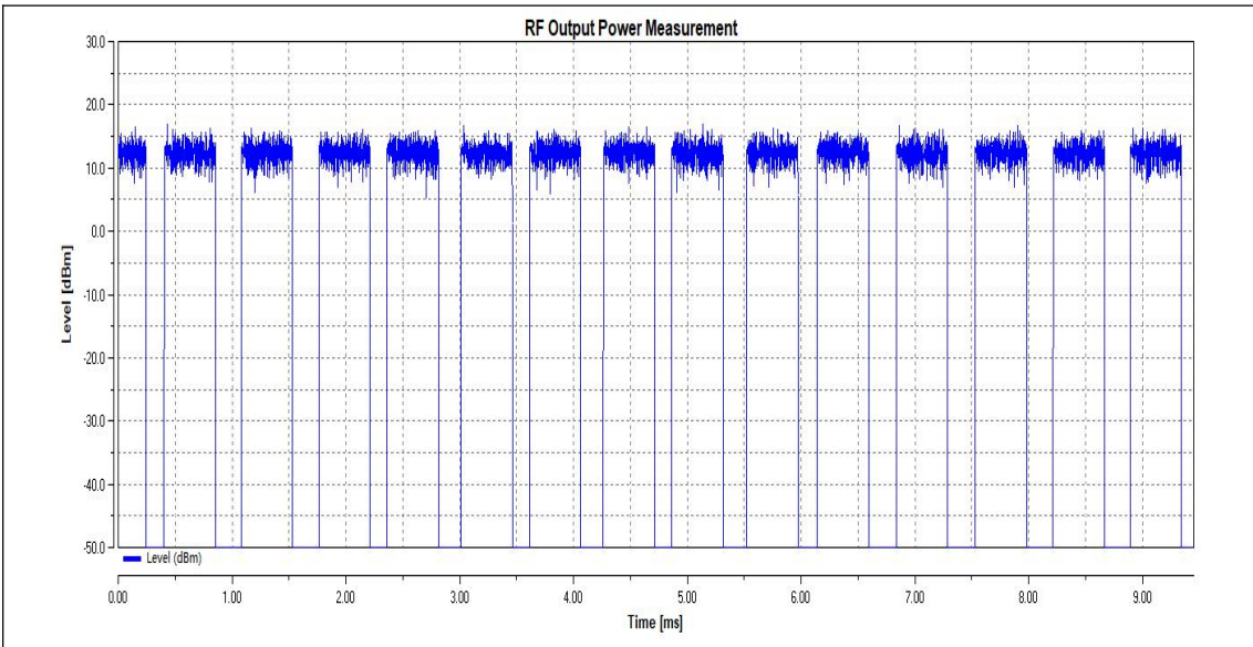
NTNV_11AX40SISO_Ant1_2422
