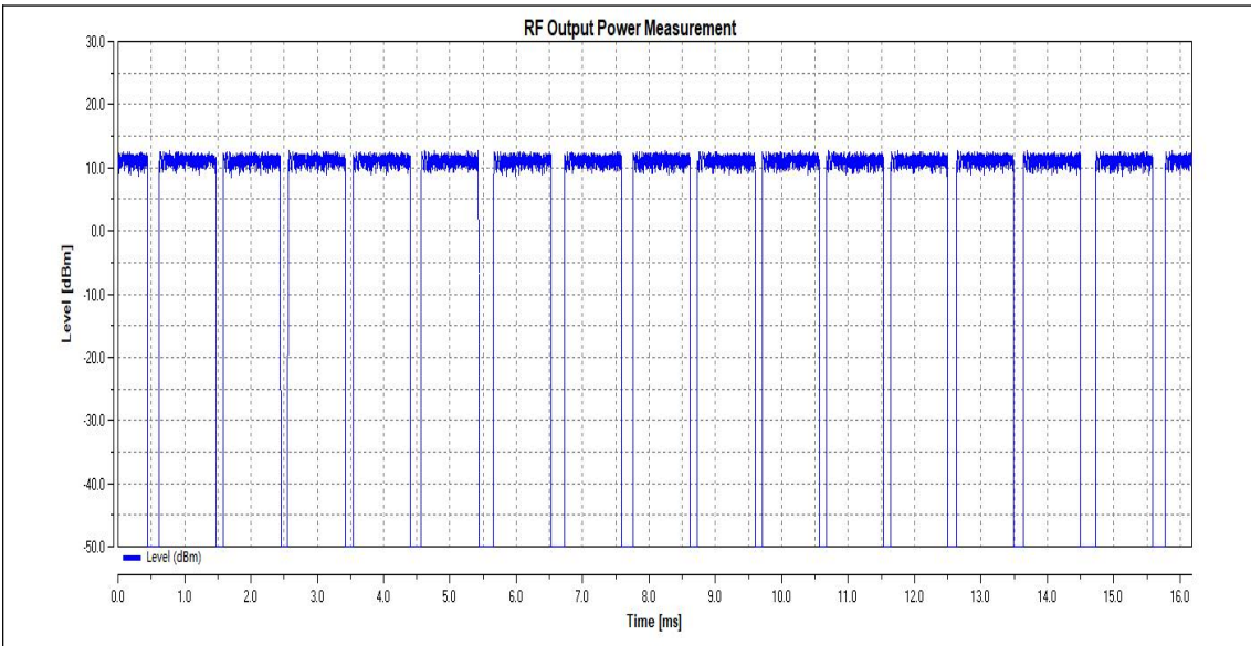
LTNV_11G_Ant1_2412
