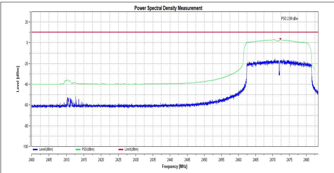
11AX40SISO_Ant1_2422
