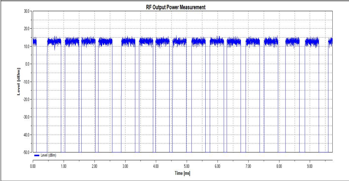
HTNV_11B_Ant1_2412
