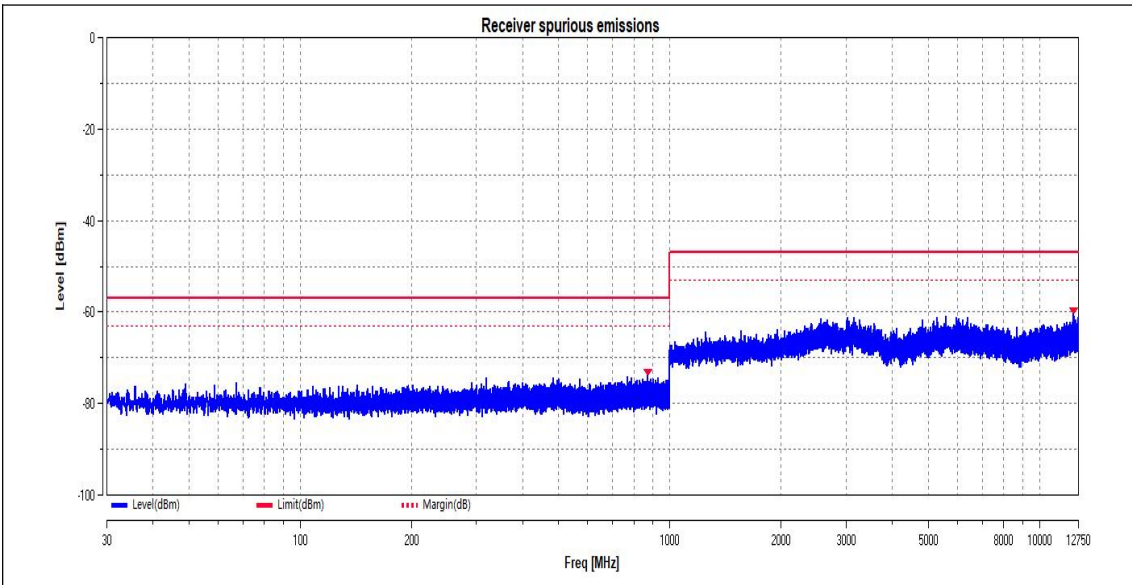
11AX20SISO_Ant1_2472
