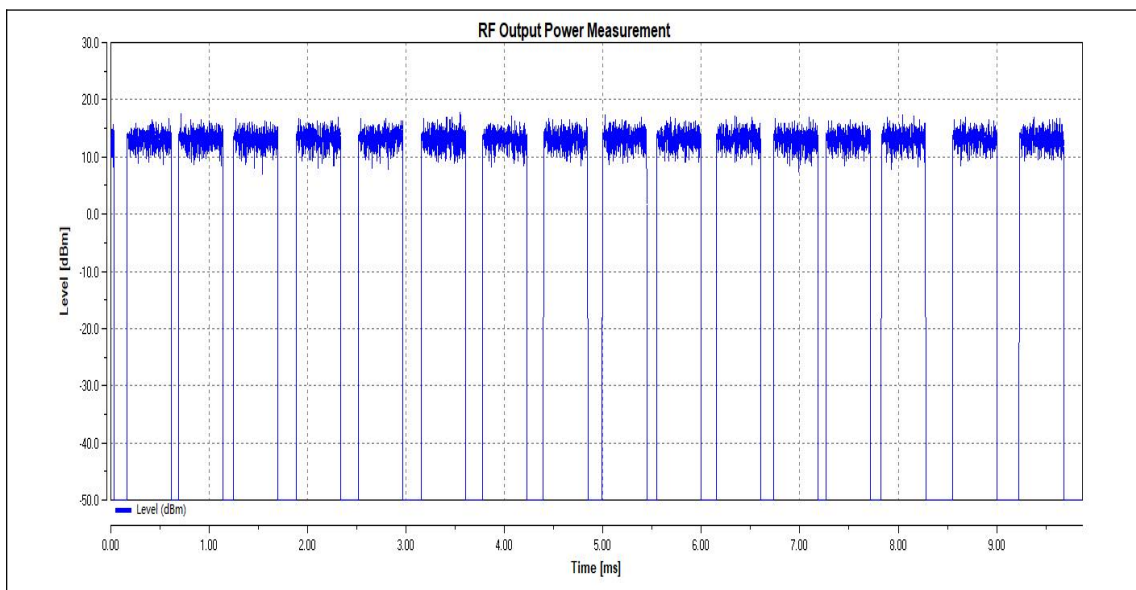
NTNV_11AX20SISO_Ant1_2442
