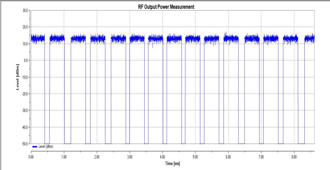
HTNV_11AX40SISO_Ant1_2442
