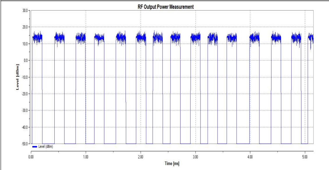
LTNV_11G_Ant1_2442
