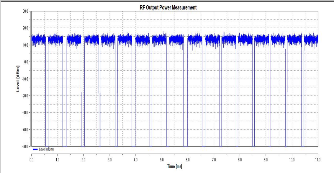
HTNV_11N20SISO_Ant1_2472
