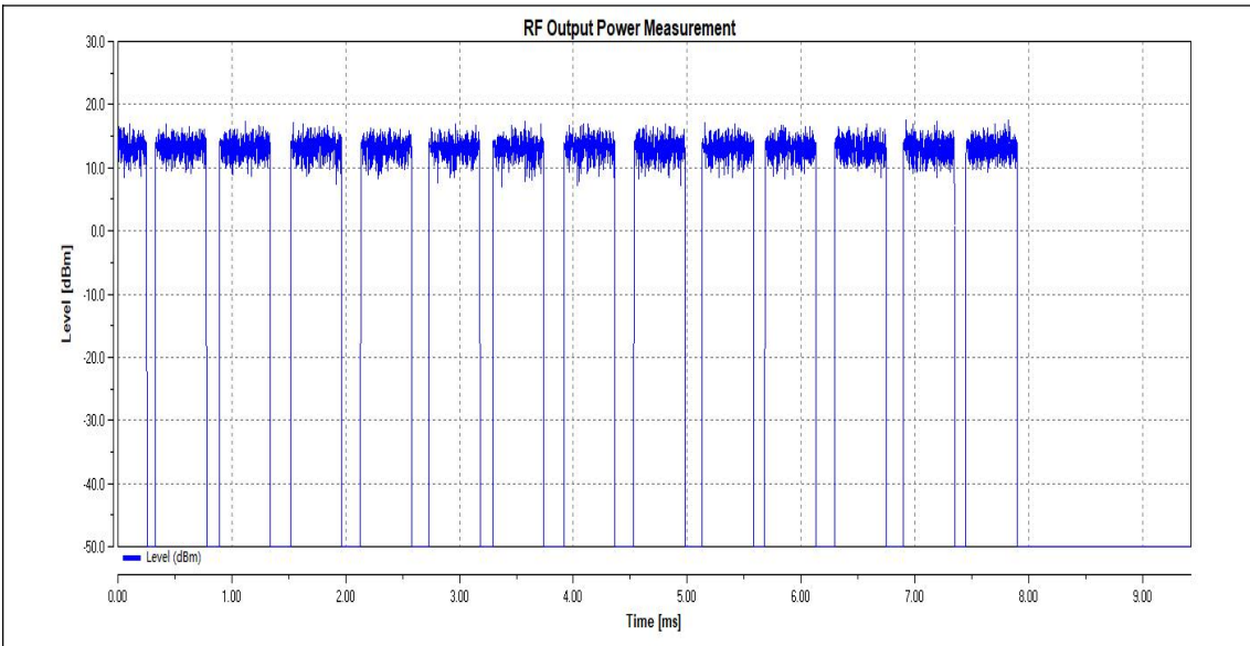
LTNV_11AX20SISO_Ant1_2442
