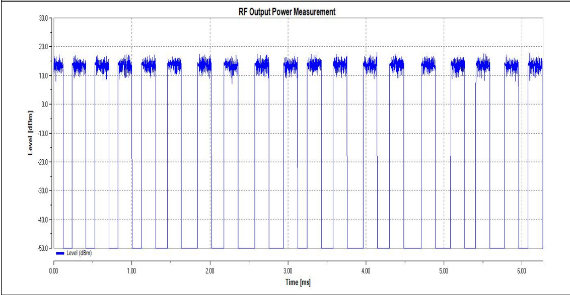
NTVN_11G_Ant1_2442
