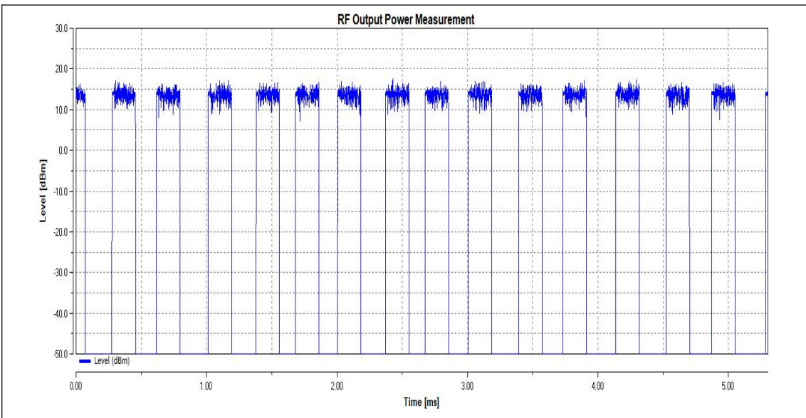
NTVN_11G_Ant1_2472
