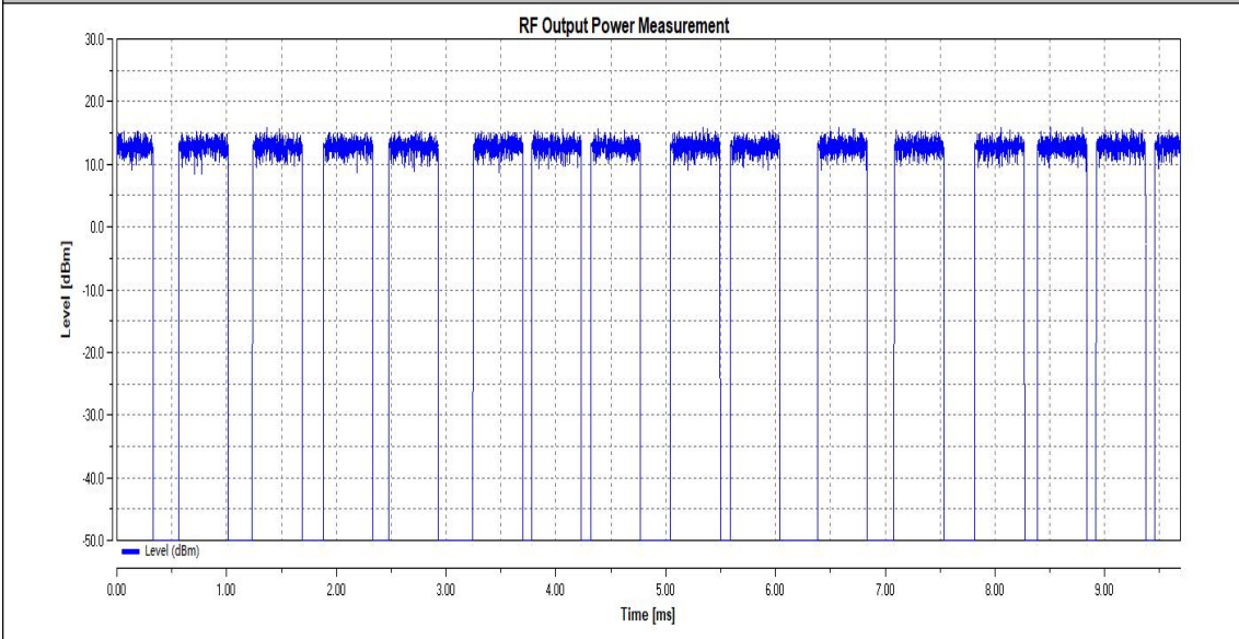
LTNV_11B_Ant1_2412
