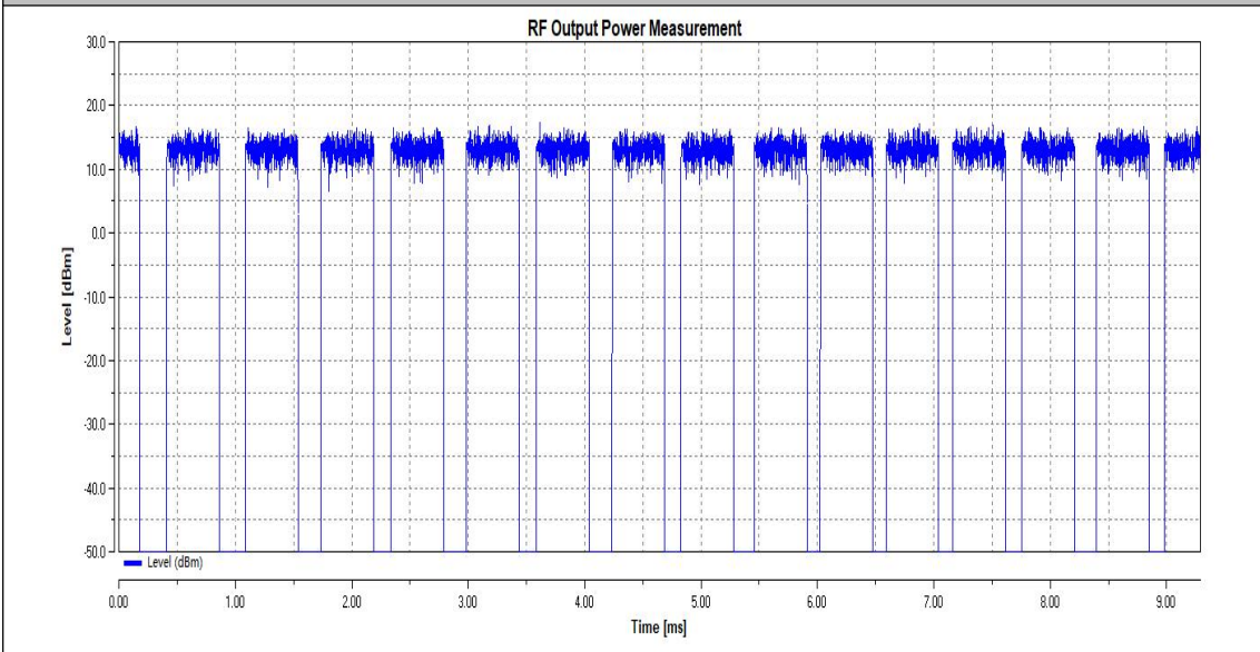
HTNV_11AX20SISO_Ant1_2472
